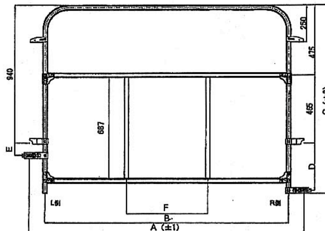
構造図
