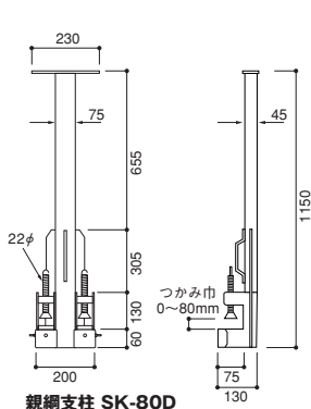
親網支柱 SK-80D
