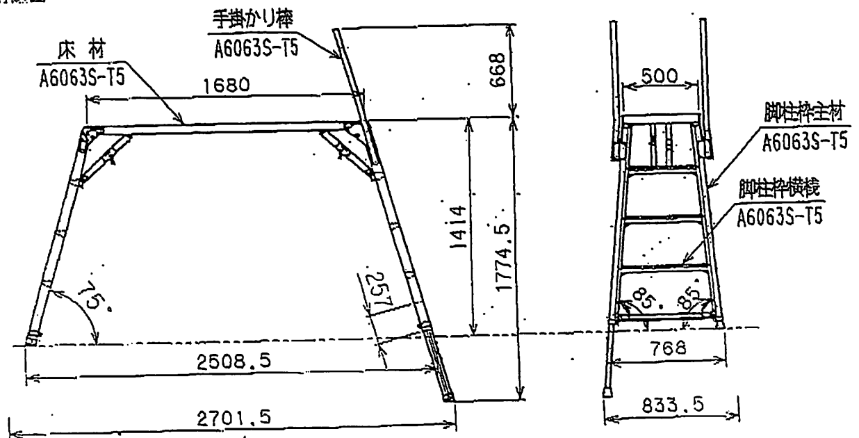
構造図
