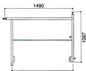
手摺枠 AHS-14W (11.2kg)
