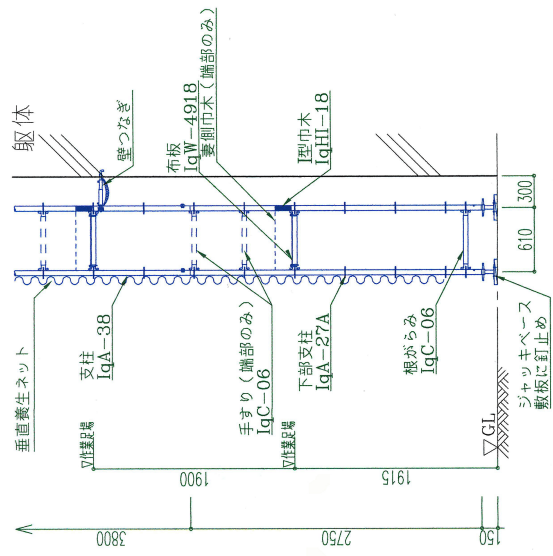
Iqシステム脚部詳細（妻側）
