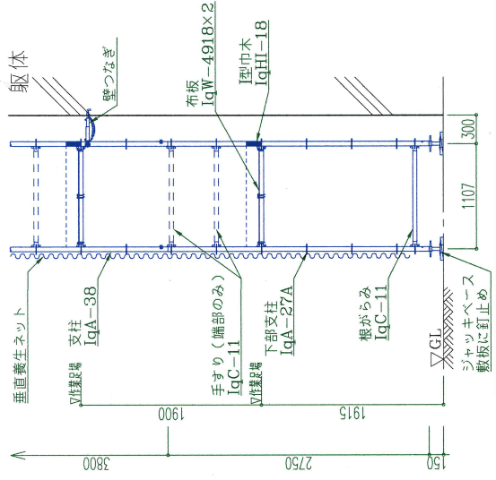
Iqシステム脚部詳細（妻側）
