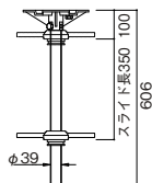
ジャッキベース ALSH-3 (5.0kg)
