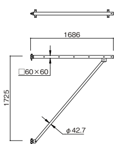
ステージ OKSHS-15 (17.8kg)
