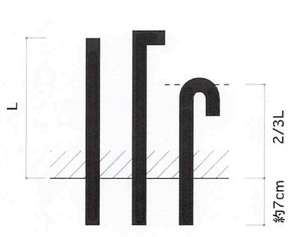
アンカーボルトの長さについて
